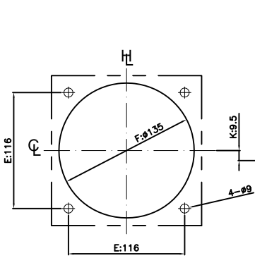
盤面孔位
