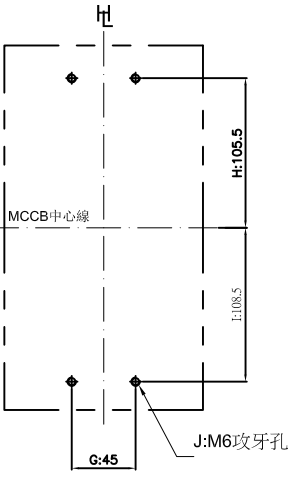
MCCB固定孔
