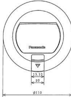
圓型地板彈插座(DU6145PF)
