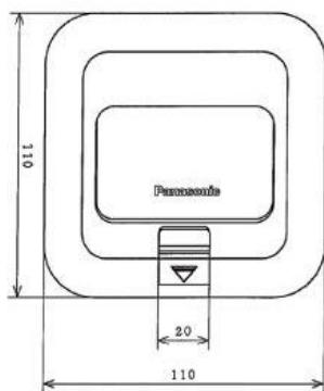
方型地板彈插座(DU6345PF)
