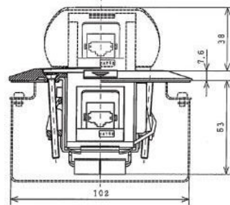
圓型地板彈插座(DU6145PF)
