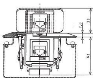
方型地板彈插座(DU6345PF)
