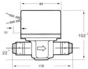
FLARE
