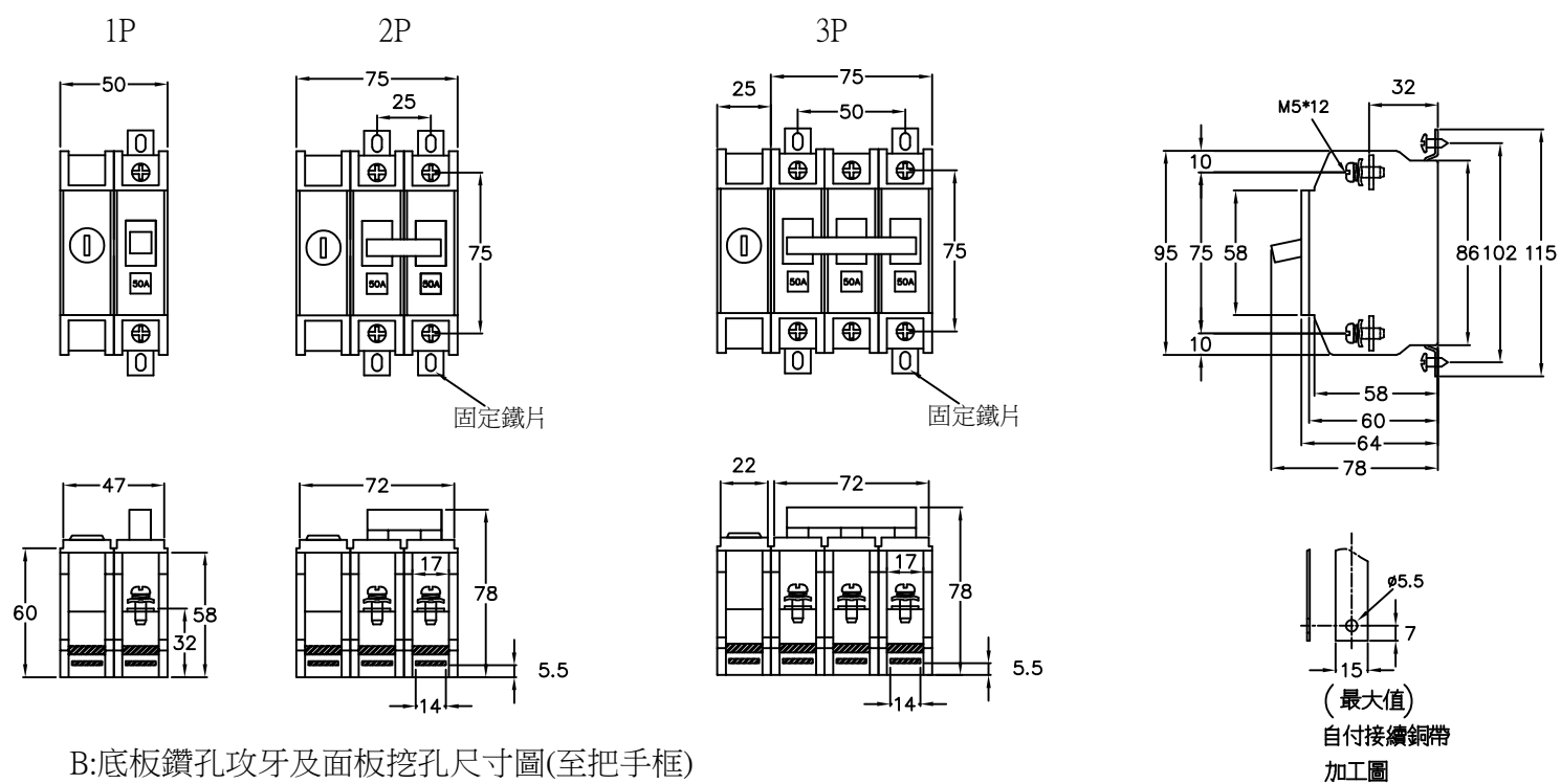
A:外型尺寸圖
