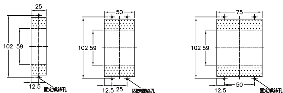
B:底板鑽孔攻牙及面板挖孔尺寸圖(至把手框)
